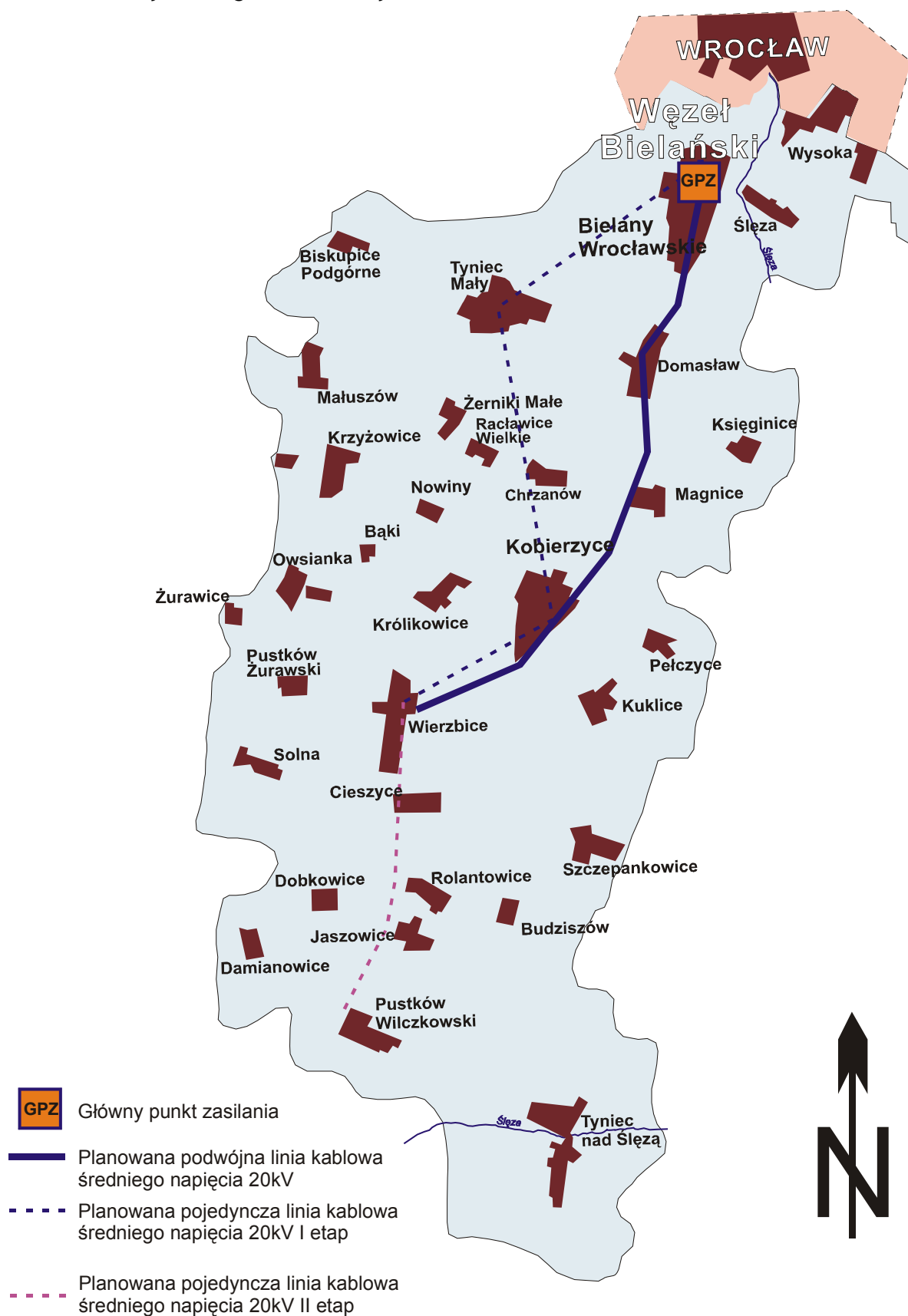
Mapa 7-4 Sieć elektryczna w gminie Kobierzyce
