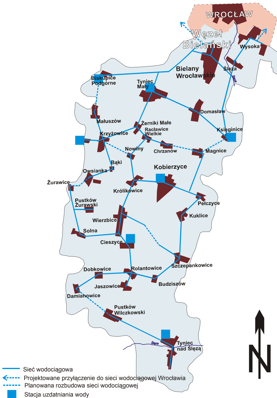
Mapa 7-1 Sieć wodociągowa w gminie Kobierzyce
