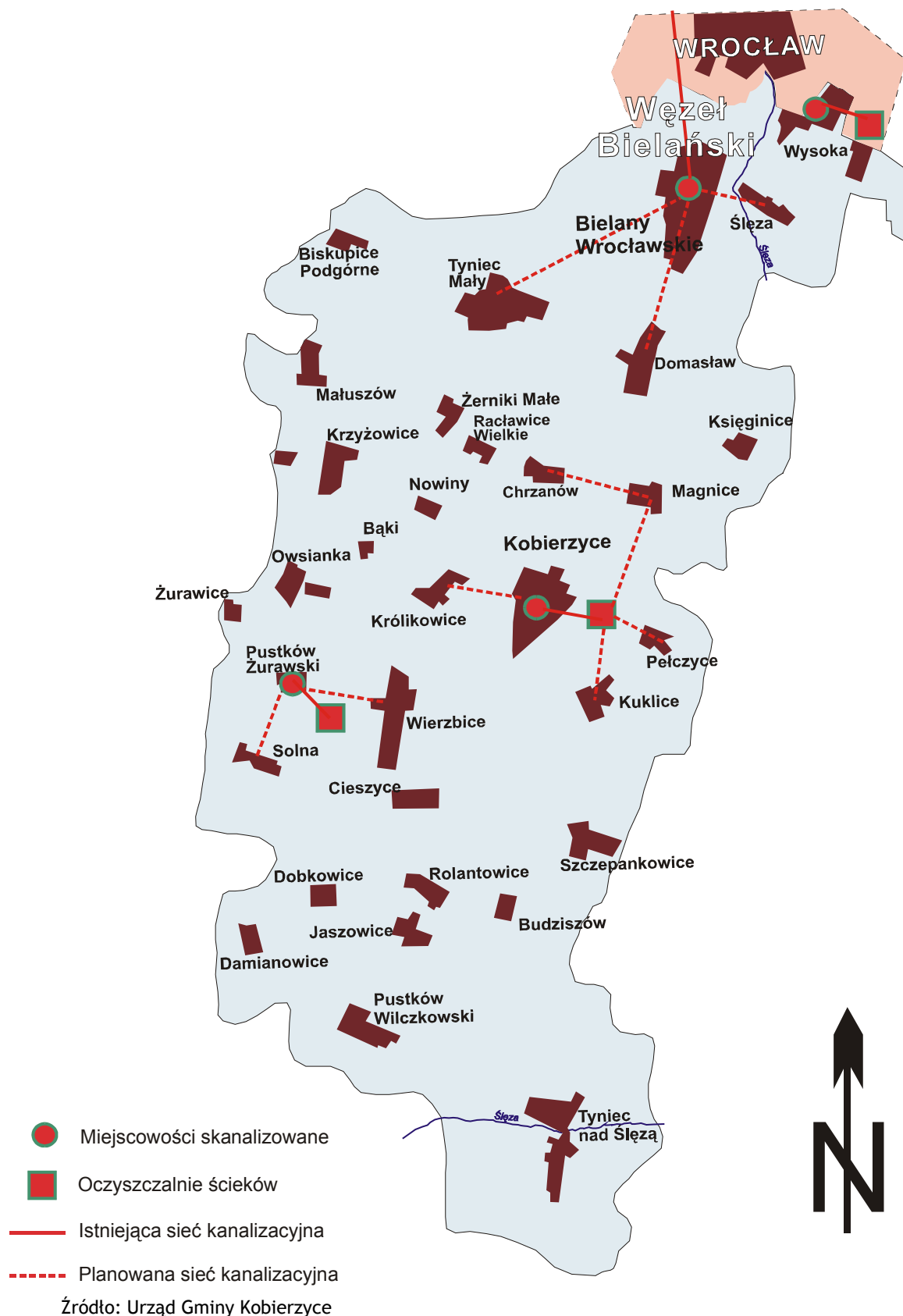
Mapa 7-3 Sieć kanalizacyjna w gminie Kobierzyce
