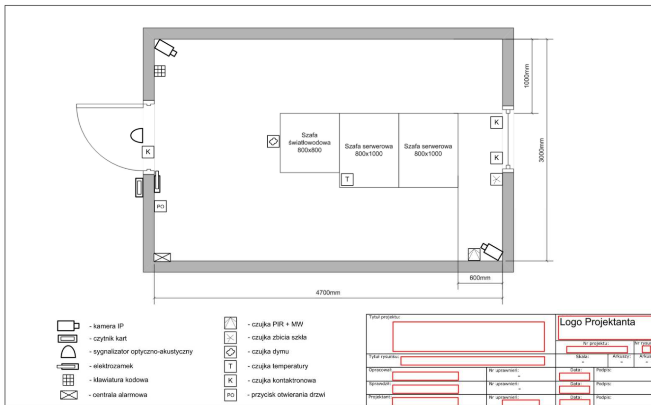
Rysunek 14. Wzór graficznej prezentacji urządzeń Zintegrowanego Systemu Nadzoru
